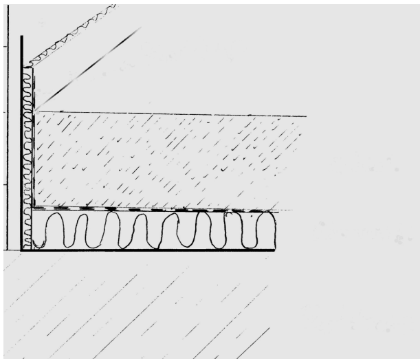
Bild 1: Handskizze Randfuge
