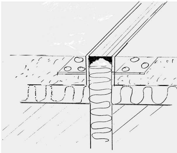
Bild 3: Handskizze Bewegungsfuge Bauwerksfuge
